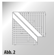
Abb. 2 Gehrungsecke [75-120°] für Querrost
