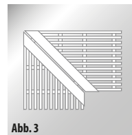
Abb. 3 Gehrungsecke [75-120°] für Parallelrost
